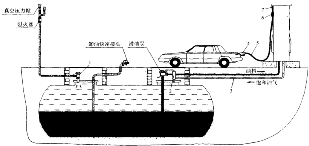
图 2 第二阶段油气回收系统示意图 1—油气回收快速接头;2—真空泵;3—油气回收管;4—油气回收油枪;5—同轴胶管;6—胶管脱离器;7—油气分离转换接头
