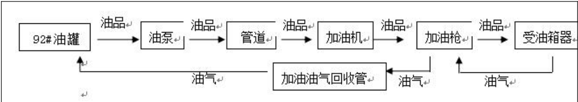
图 2.5-1 汽油加油工艺流程图
