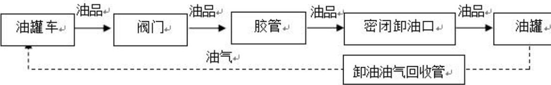
图 2.2-3 汽油卸油工艺流程图
