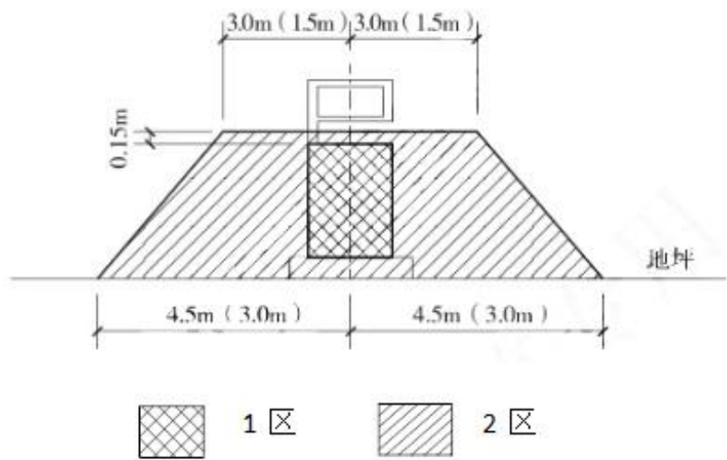
图3.9-2汽油加油机爆炸危险区域划分
