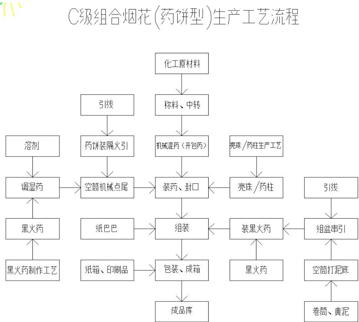
图 2-1：组合烟花类生产工艺流程图
