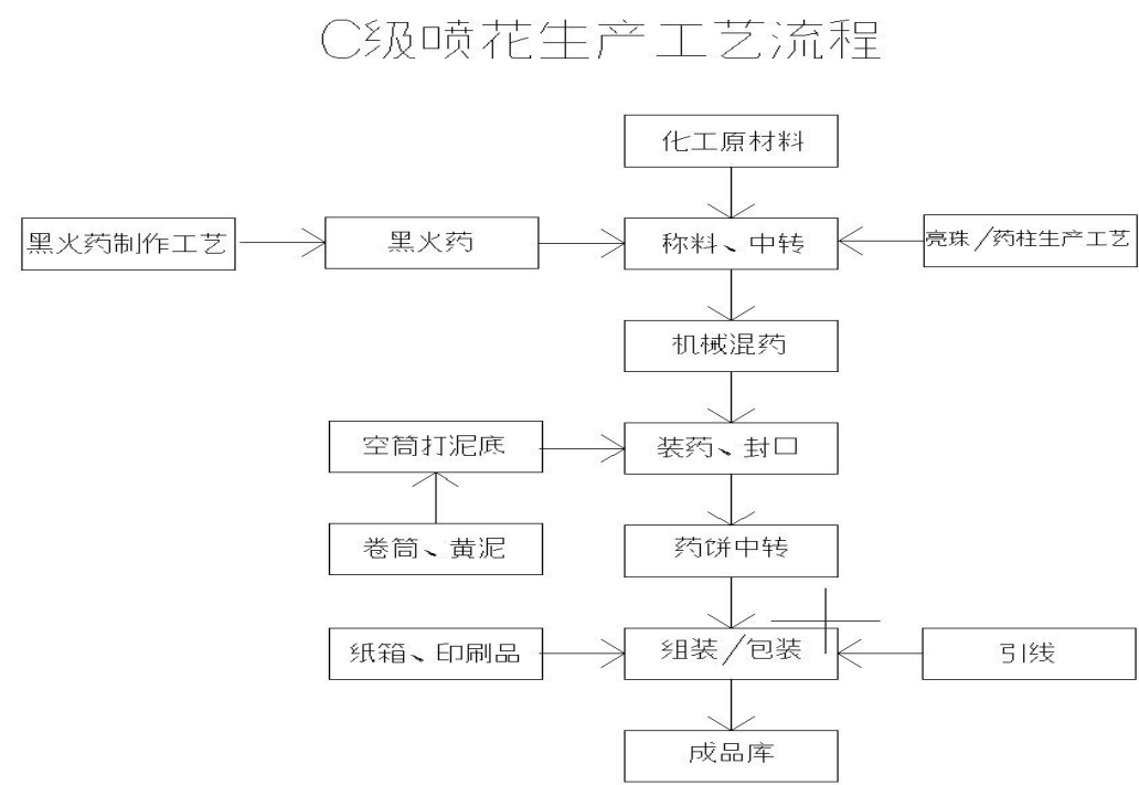
图 2-2：喷花类生产工艺流程图
