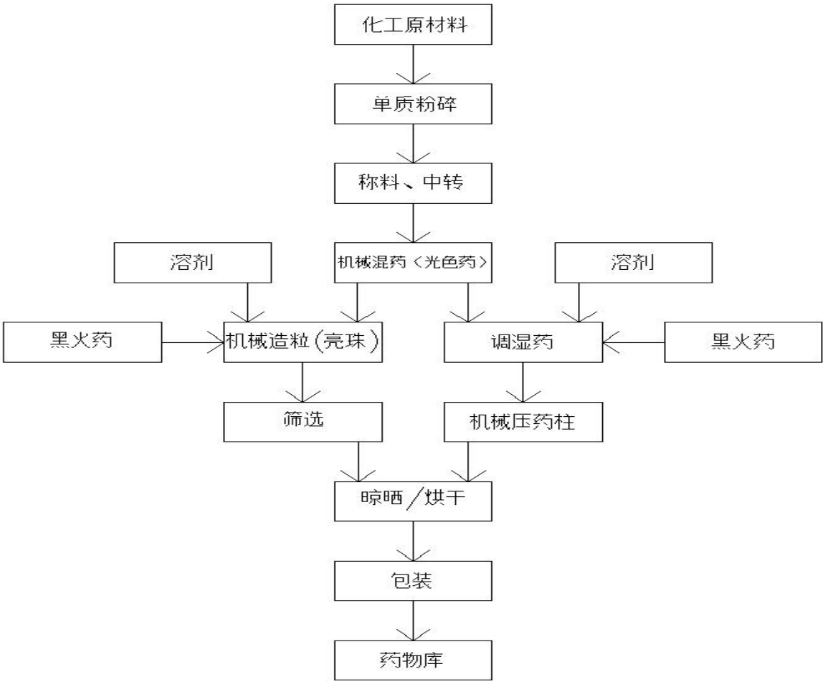
图 2-5：烟花药（亮珠/药柱）生产工艺流程图
