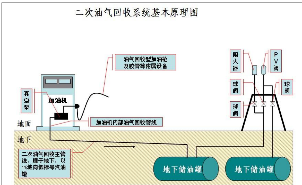
图 2.2-5 二次油气回收系统基本原理图
