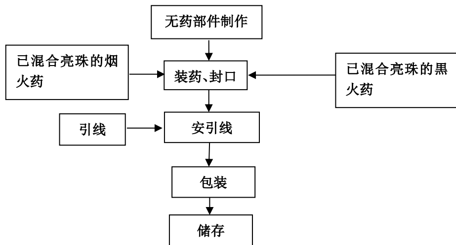
图 2-4-3 喷花类生产工艺流程图
