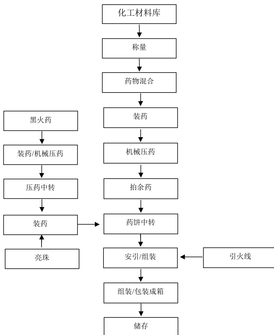
图 2-2：升空类（火箭）生产工艺流程图
