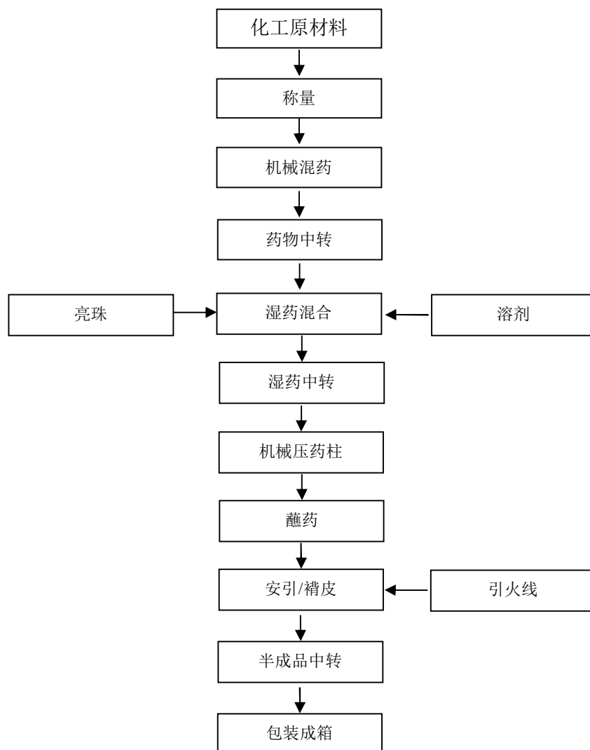
图 2-3：玩具类（玩具造型）生产工艺流程图
