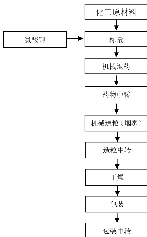
图 2-4：烟雾效果件生产工艺流程图
